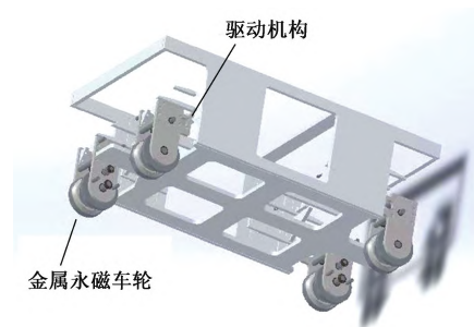
图 1 爬壁机器人机械结构
